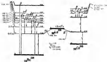
צור 10. תיאור דיאגרמטי של התפרקות \beta^- ו \beta^+ (עם סיכויים 70% בהתאמה) של גרעין ^{138}\text{La} (ע"פ NDS, ר' ביכלר)
